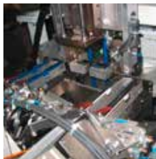
Zuführsystem Schreibgerätemontage
